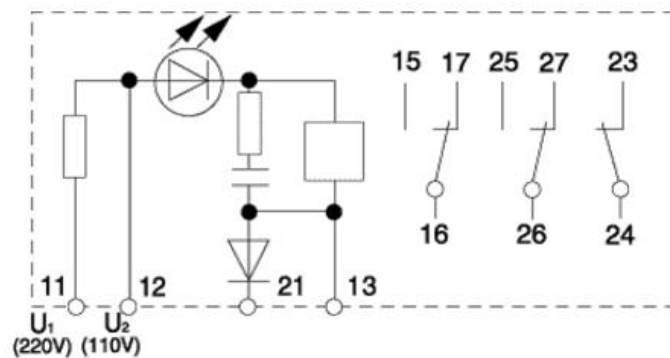
接线图
