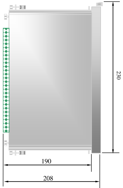
侧视图
