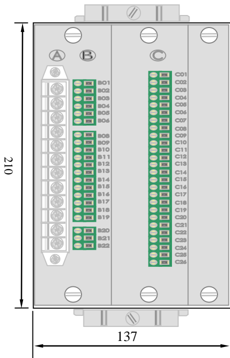
正视图
